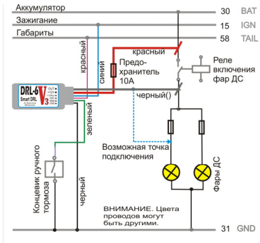
Рис. 1. Подключение DRL-6-V3 с управлением фарами дальнего света ДС параллельно силовым контактам «Реле включения фар ДС» - подачи «+12В». В некоторых автомобилях цепь 15 может обозначаться как «X» или «IGN».
