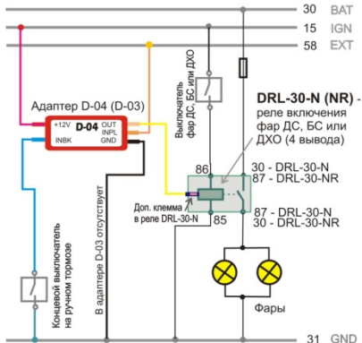
Рис. 1. Подключение DRL-30-N (NR) для управления фарами ДС, БС или светодиодных ДХО с обеспечением «Режима ДХО». Типовое подключение: управление - подачей +12В на обмотку, силовая цель - подача +12В в нагрузку. ВНИМАНИЕ! Вход INPL адаптера D-03 должен быть обязательно подключен. При упрощенном подключении на доп.клемму подается только +12В от цепи «15 Ignition» («+12В Зажигание»)
