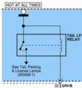
Рис. 8. Подключение реле с объединенными цепями силовых контактов и обмотки.
