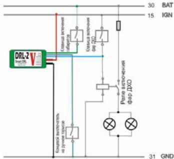
Рис. 1. Подключение DRL-2-V с управлением силовым реле «Реле включения фар ДХО» подачей «+12В». В автомобилях ВАЗ цепь 15 может обозначаться как «Х».
