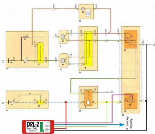
Рис. 4. Подключение контроллера DRL-2-L в автомобиле Hyundai Accent.
