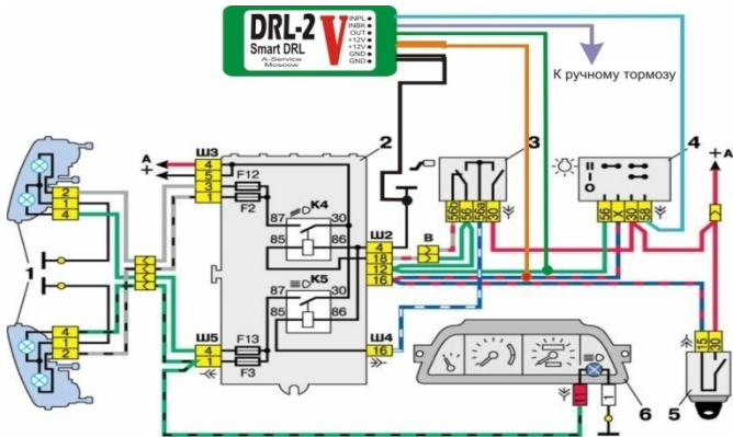
1 – блокфары, 2 – монтажный блок, 3 – подрулевой переключатель, 4 - переключатель наружного освещения, 5 – замок зажигания, 6 – приборная панель.
