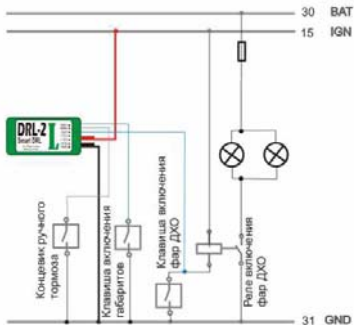
Рис. 2. Подключение DRL-2-L с управлением силовым реле «Реле включения фар ДХО» подачей «минуса» («массы»)
